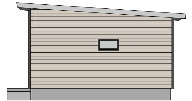
Julkisivu 2 1:100
