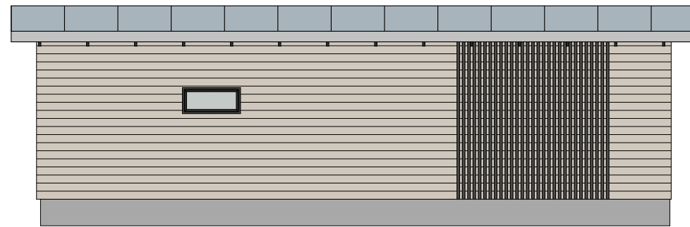
Julkisivu 3 1:100
