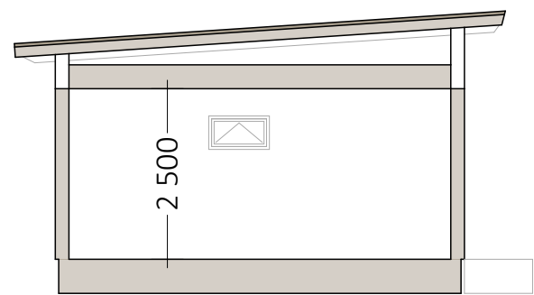
Leikkaus 1:100
